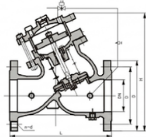
PISTON TYPE
